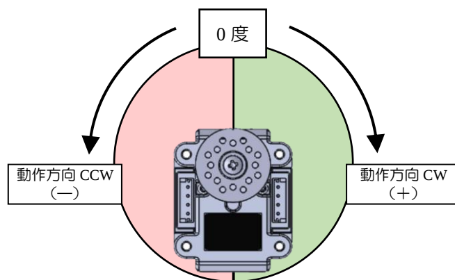
Fig. 2.9 角度の定義
