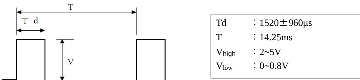
Fig. 3.1 PWM 信号の仕様
