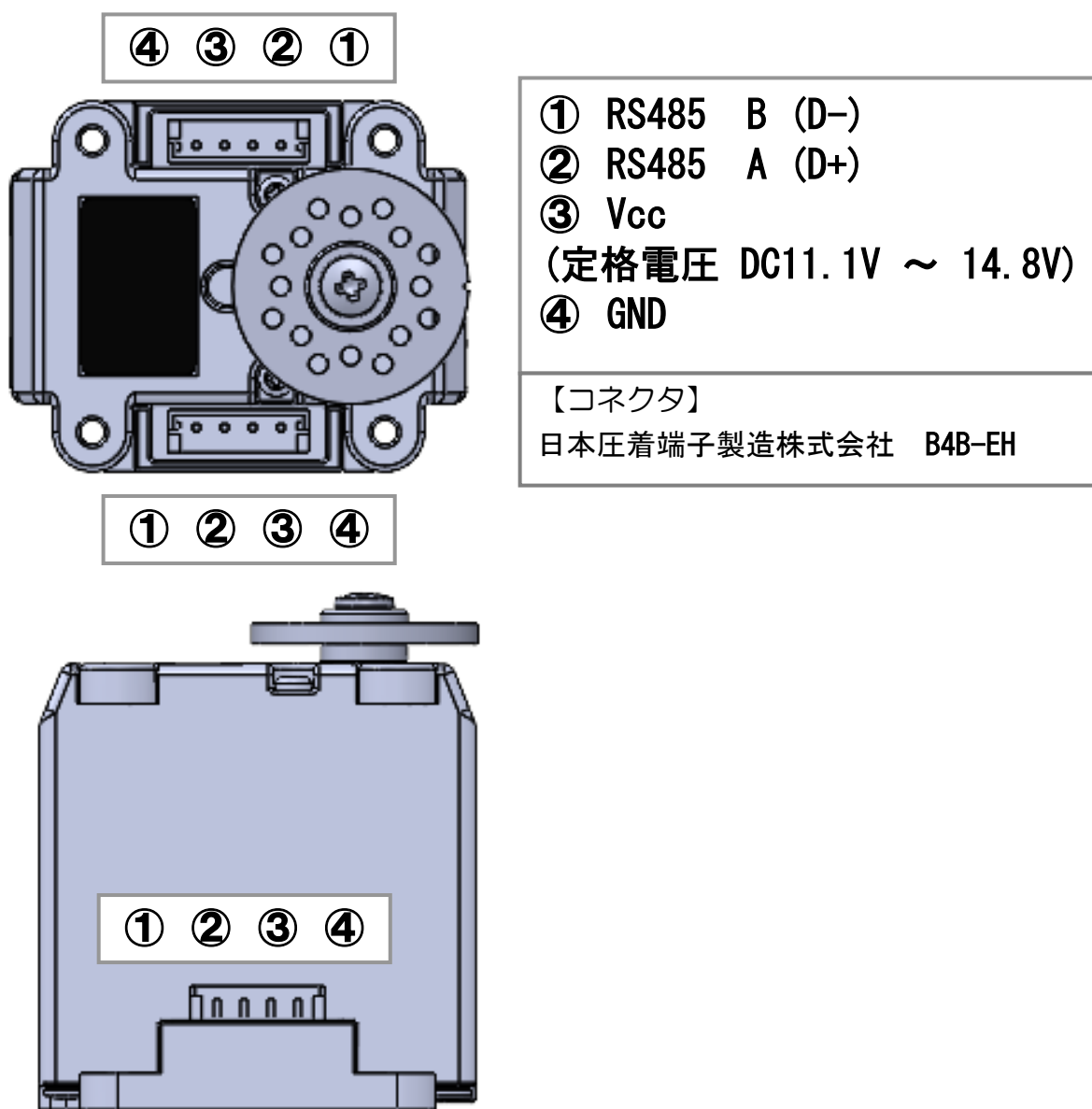
Fig. 2.5 コネクタピン配置
