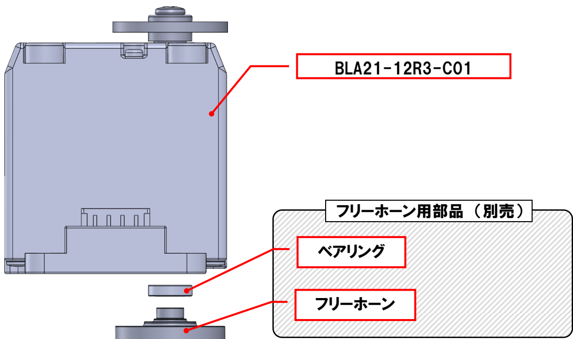
Fig. 2.1 反対軸構成（イメージ図）
