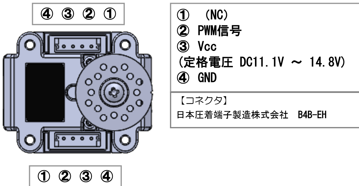
Fig. 2.6 コネクタピン配置
