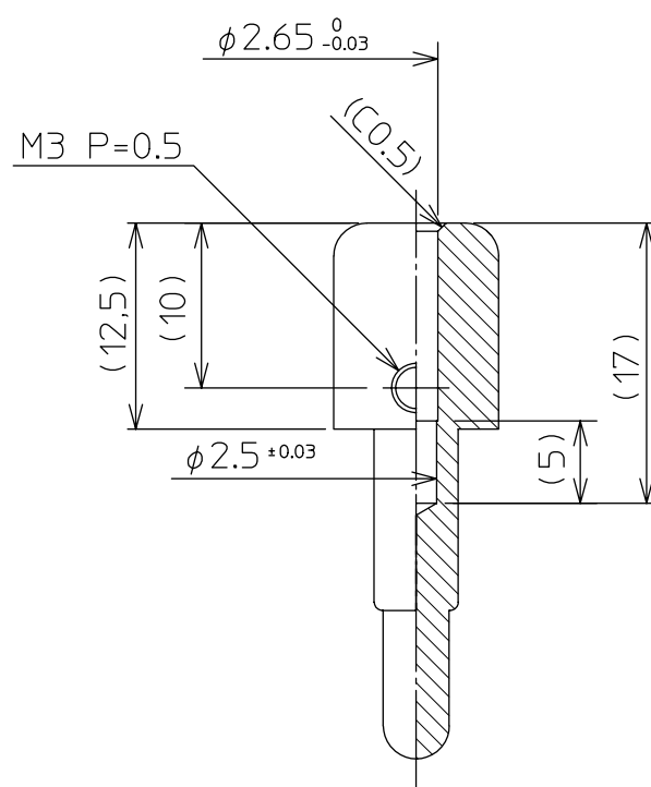
エレメント挿入穴 詳細図 (尺度2/1)
